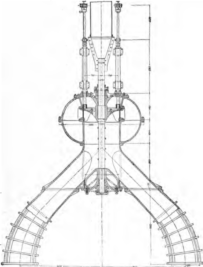
Fig. 44. Schnitt durch die Biagaraturbinen.
